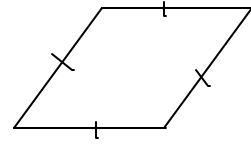
rhombus
