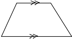
trapezium
