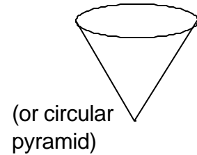
cone
